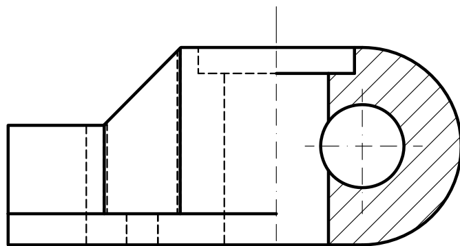
SECCIÓN A-A
